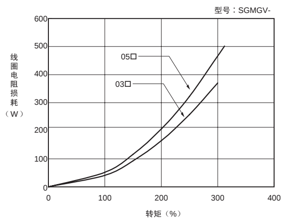
(d) 旋转型伺服电机 SGMGV 型
