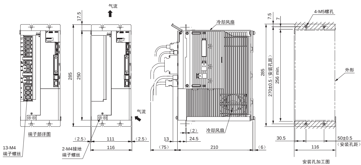
(8) 三相 AC 200V SGD V-330A□□A001
