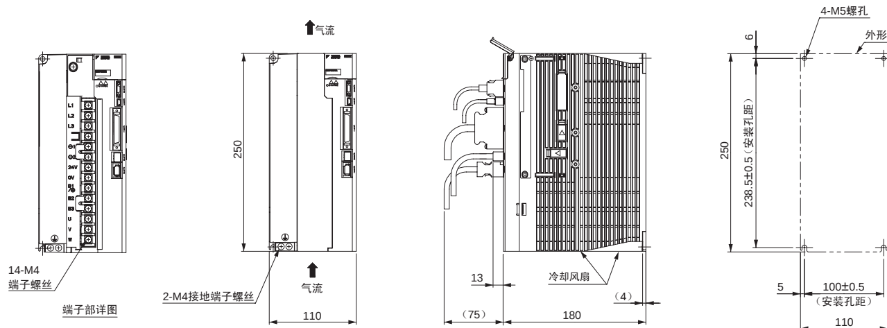
(12) 三相 AC 400V SGD V-8R4D□□A, -120D□□A
