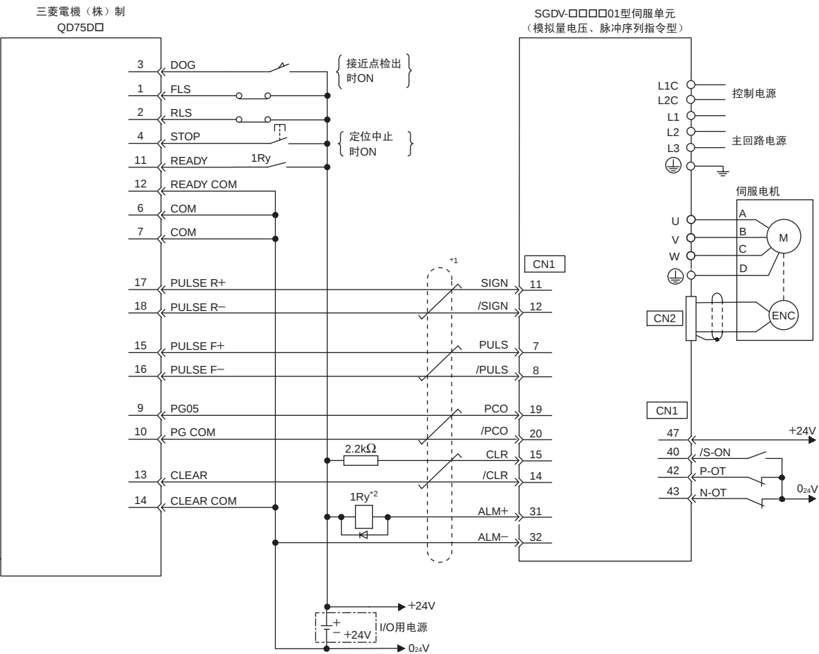
与三菱電機（株）制定位装置QD75D□的连接示例（位置控制）
