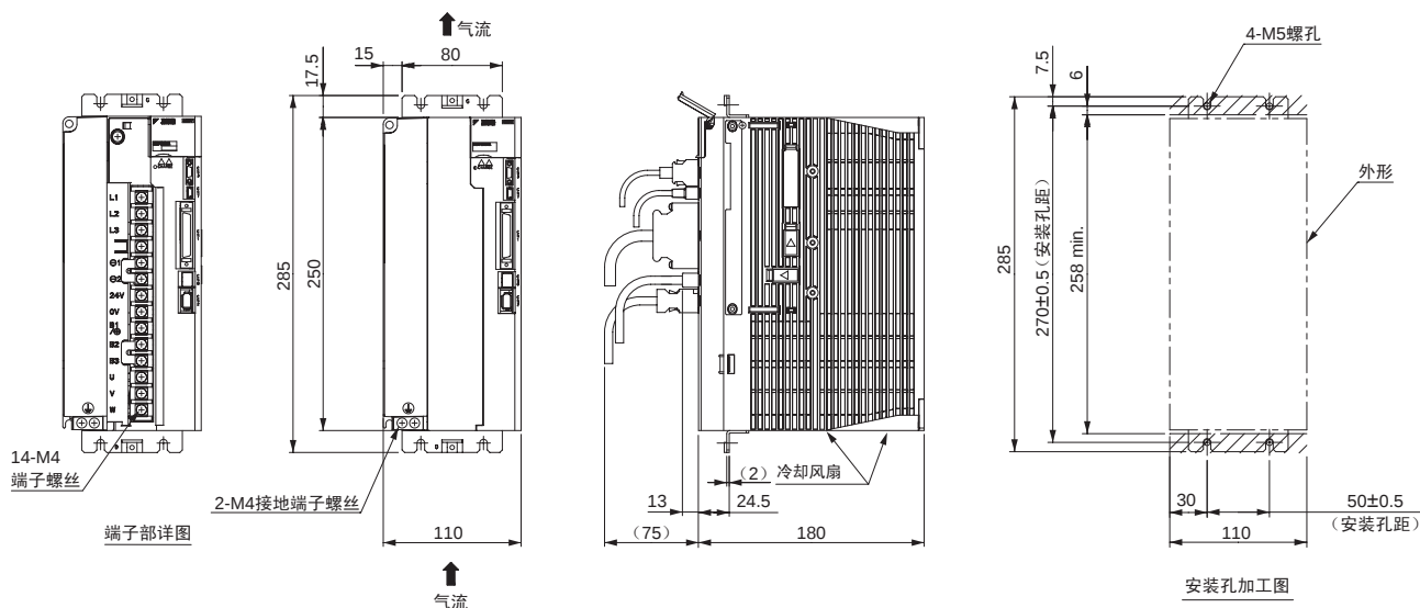
(12) 三相 AC 400V SGD V-8R4D□□A001, -120D□□A001
