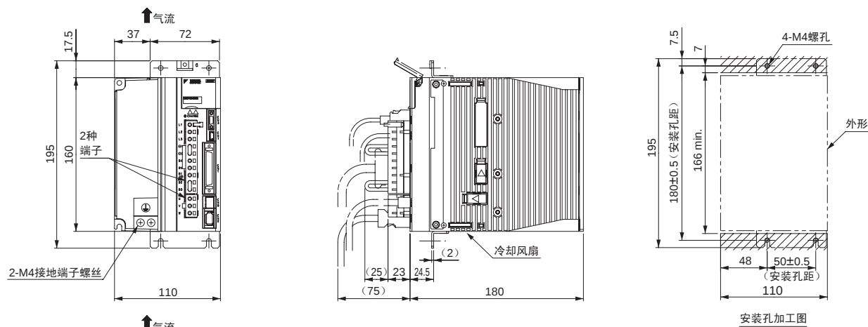
(11) 三相 AC 400V SGD V-1R9D□□A001, -3R5D□□A001, -5R4D□□A001
