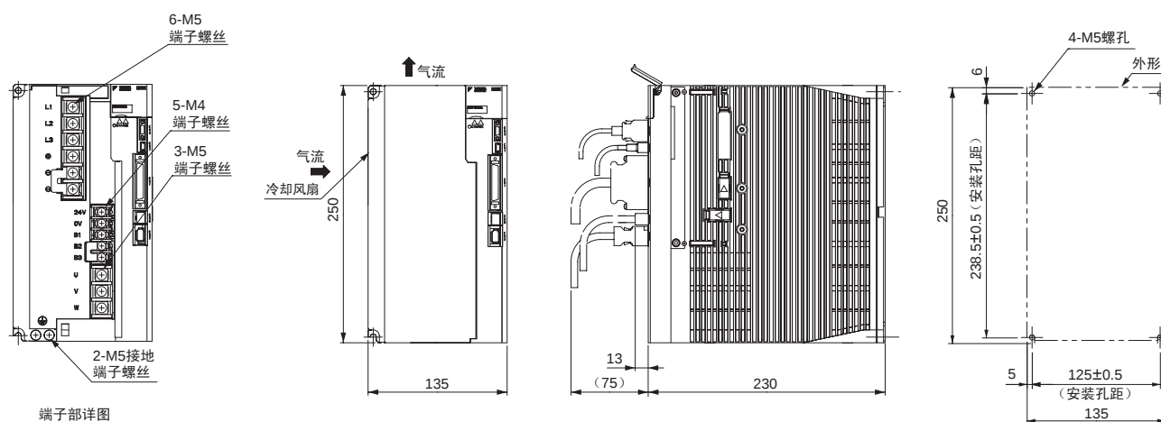
(13) 三相 AC 400V SGD V-170D□□A
