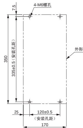
安装孔加工图
